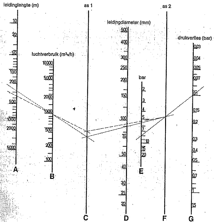
Figuur 4.5: Nomogram voor de bepaling van de leidingdiameter van een hoofdleiding.
