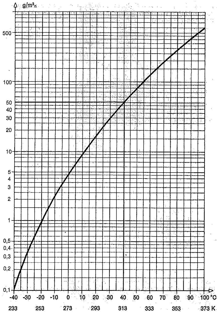
Figuur 3.27: Dauwpuntskromme.
