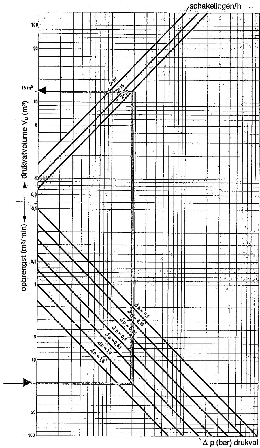
Figuur 3.32: Volumebepaling bij een drukval.
